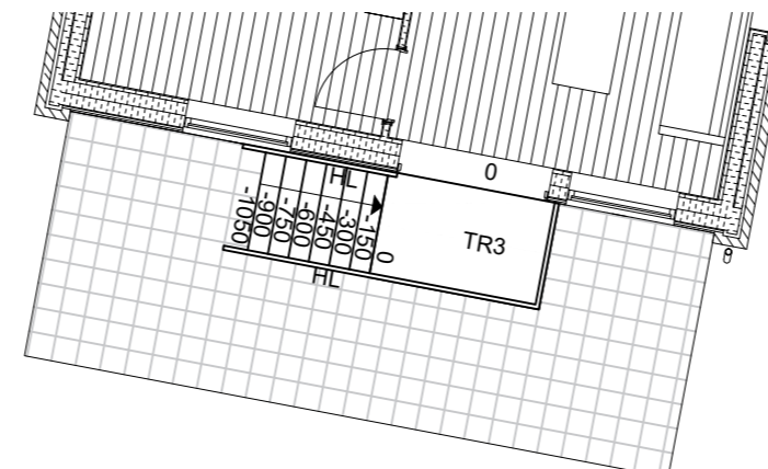
Plan 1:100, Terrænspring 451-1050 mm 19 stk
