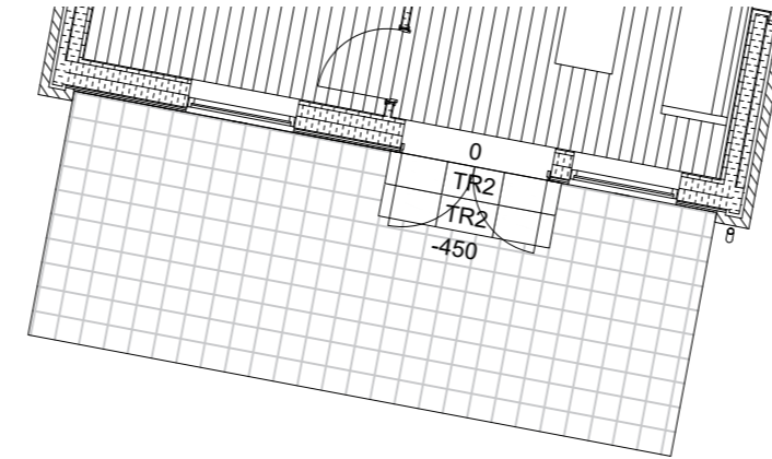
Plan 1:100, Terrænspring 301-450 mm 22 stk
