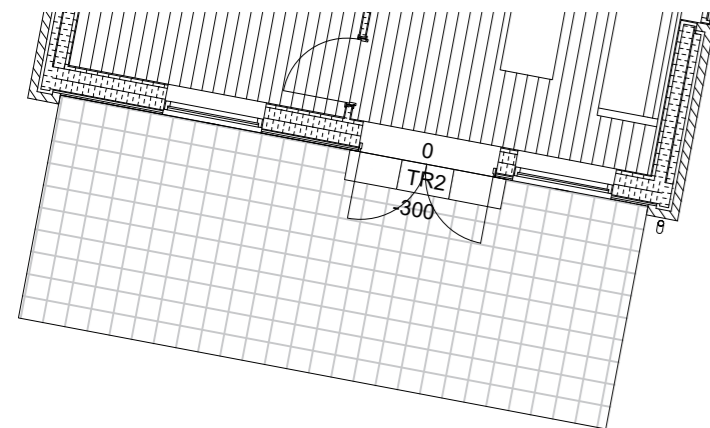
Plan 1:100, Terrænspring 151-300 mm 76 stk
