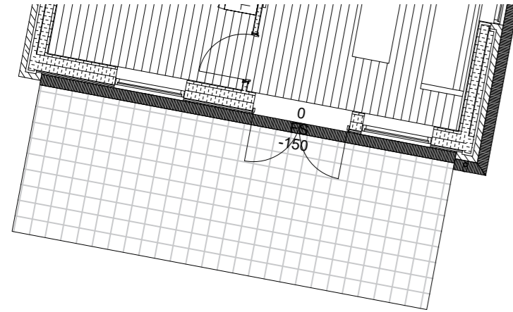
Plan 1:100, Terrænspring 0-150 mm 39 stk
